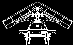
Vee Position
